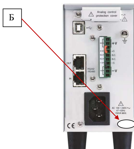
Рисунок 2 – Схема пломбировки от несанкционированного доступа (Б).
