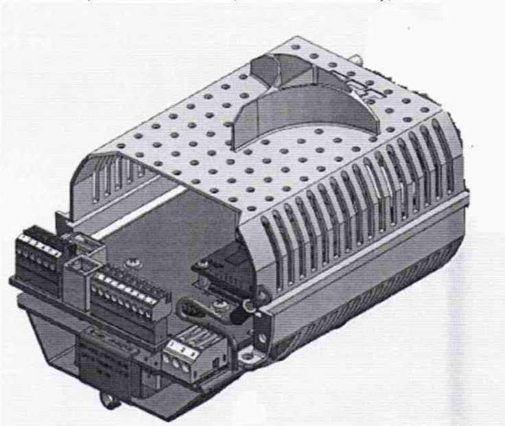
Рисунок 1 – Схема расположения плат в ЭВБ
