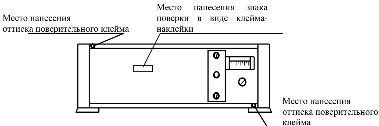
Рисунок 2 - Место нанесения оттиска поверительного клейма и знака поверки в виде клейма-наклейки на задней панели вольтметров.
