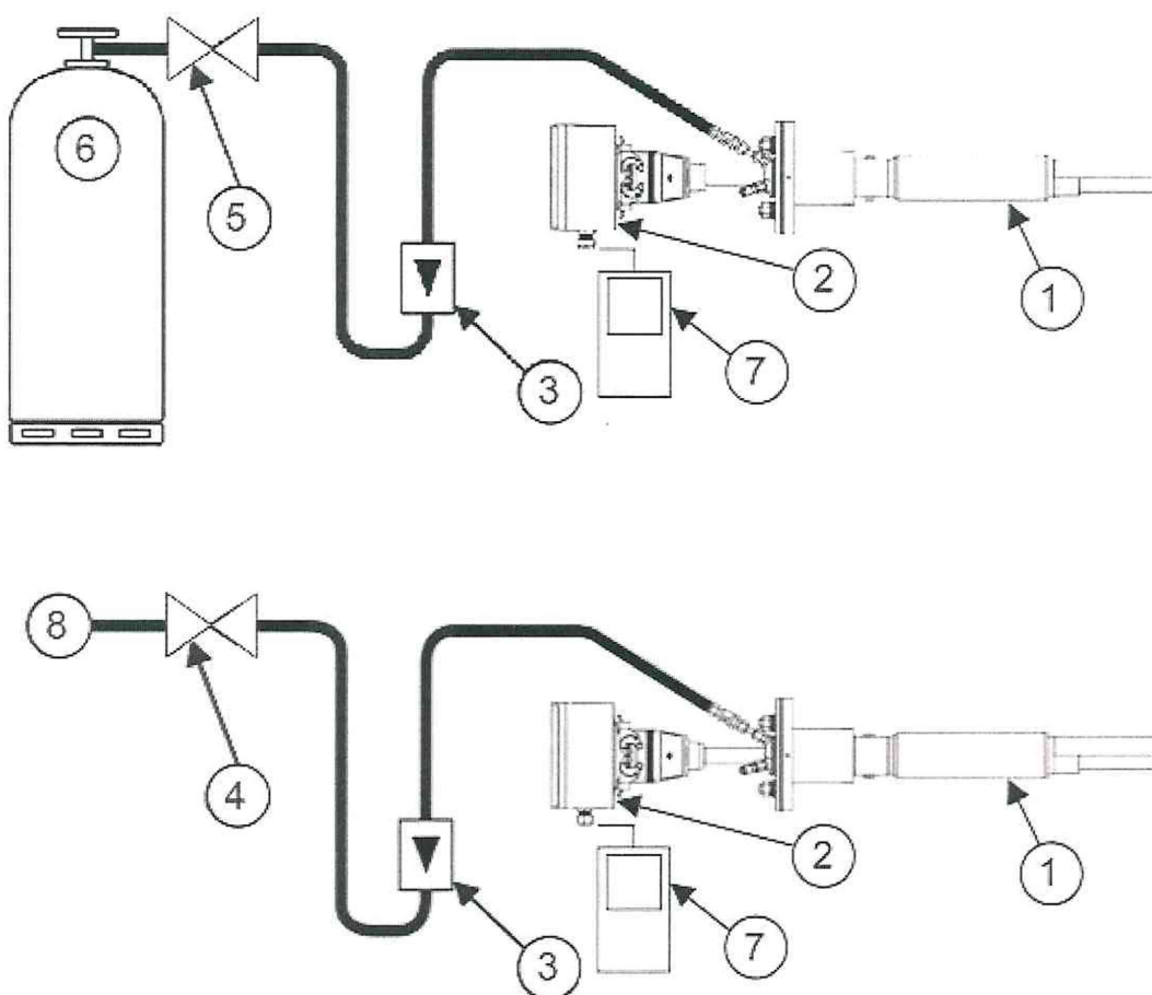
Рисунок 1 – Схема поверки газоанализатора.
