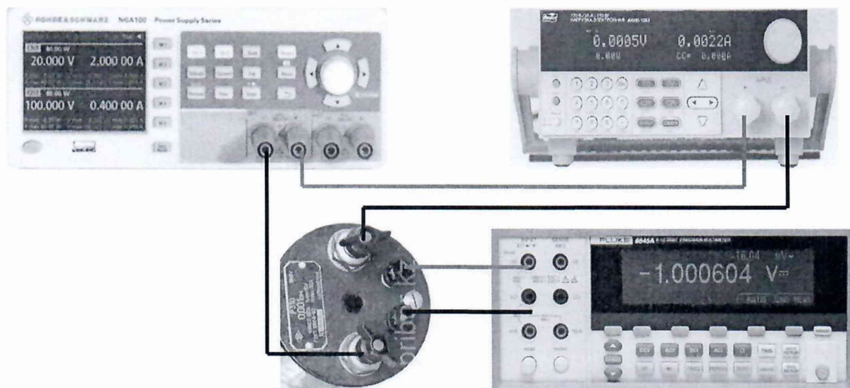
Рисунок 5 – Структурная схема соединения СИ для определения нестабильности силы постоянного тока при изменении напряжения на нагрузке от 10 % до 90 %
