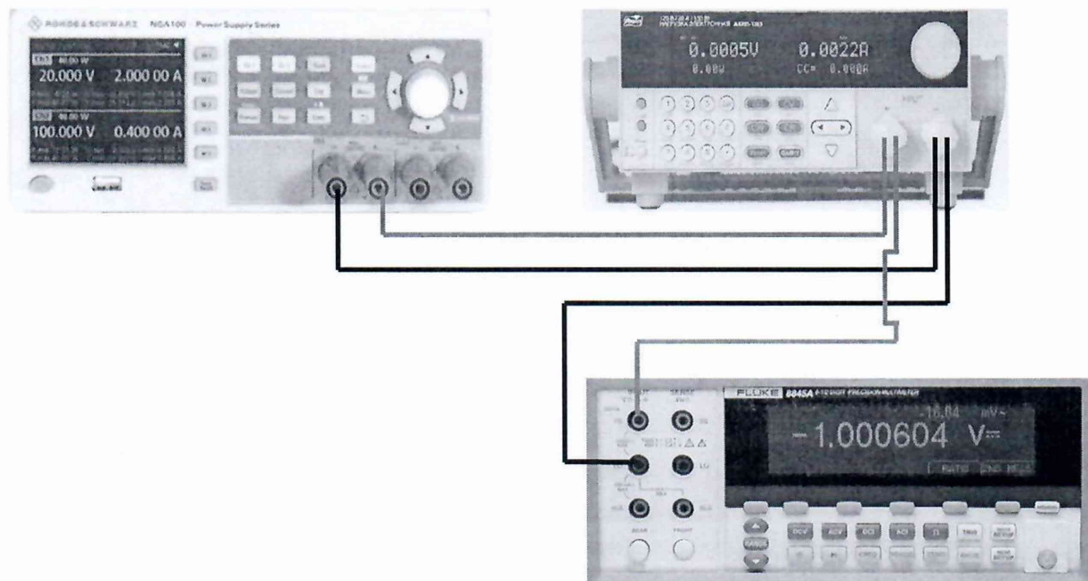
Рисунок 2 – Структурная схема соединения СИ для определения нестабильности выходного напряжения постоянного тока при изменении силы тока на нагрузке
