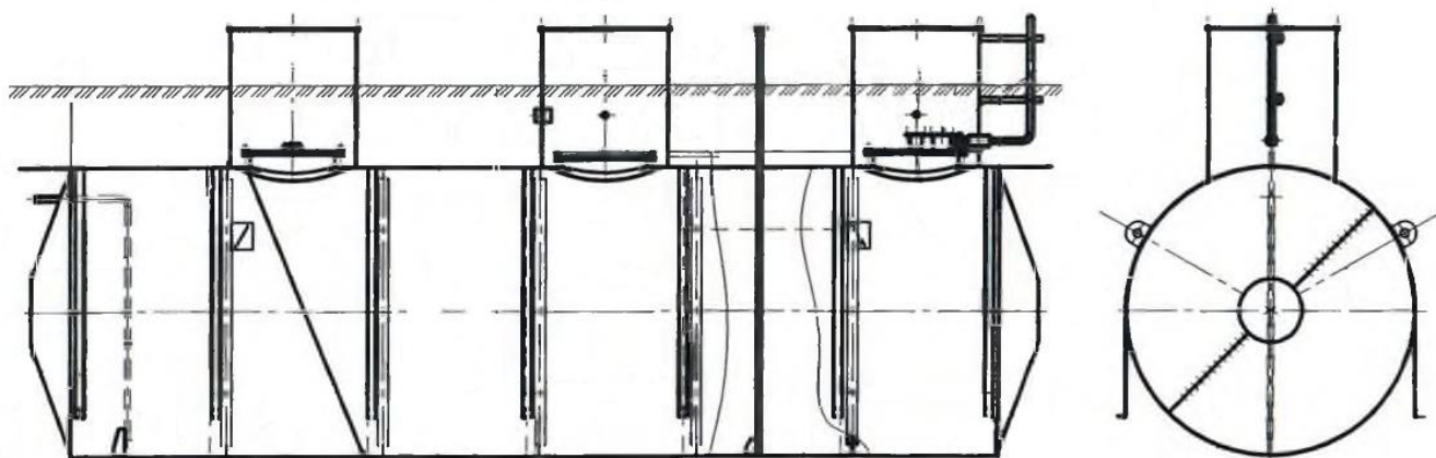
Рисунок 3 – Общий вид резервуара РГС-50
