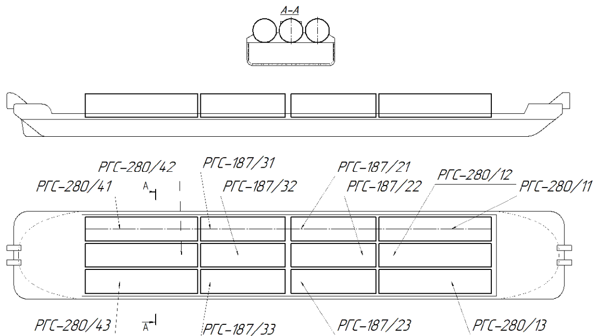
Рисунок 1 - Общий вид, номера и расположение резервуаров на барже проекта КМ16801
