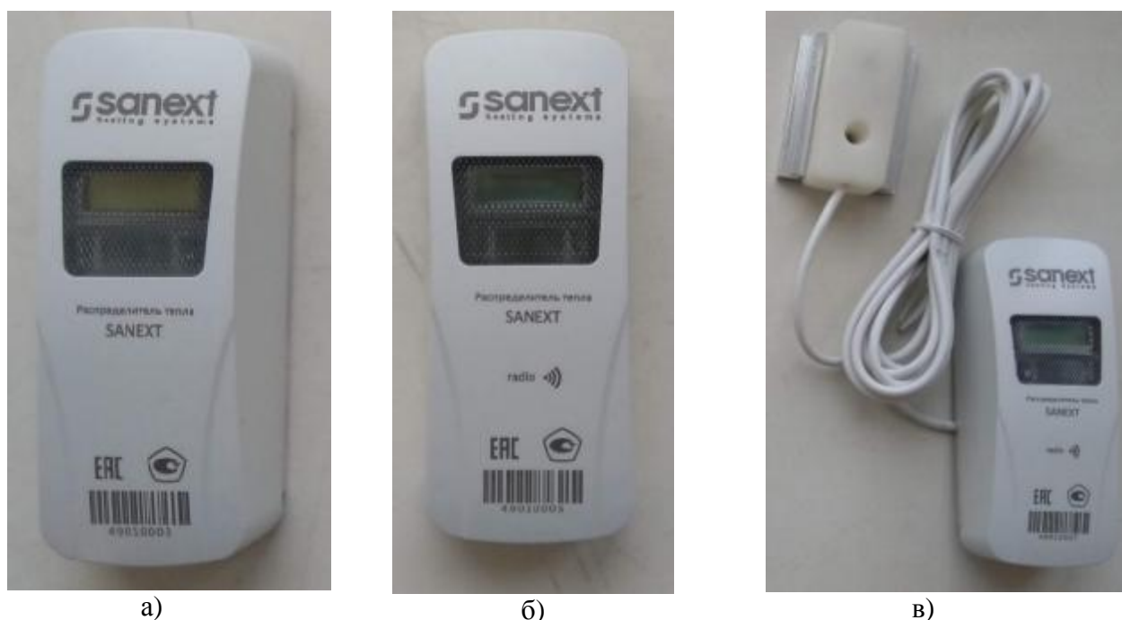
Рисунок 1 – Общий вид распределителей: а) распределитель SANEXT; б) распределитель SANEXT-R; в) распределитель SANEXT-R-V
