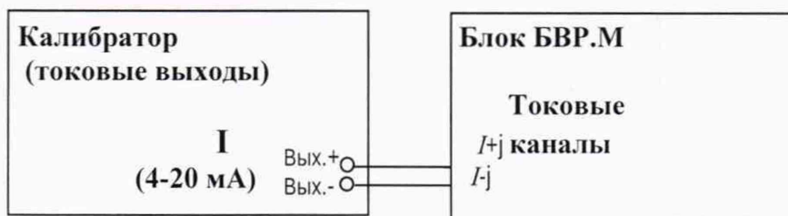
Рисунок 1 – Схема подключения СИ при определении погрешности по токовым каналам
