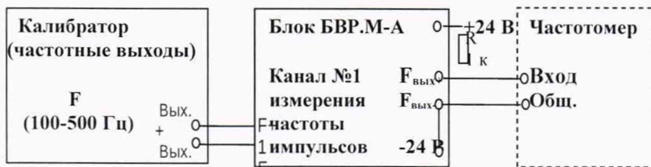
Рисунок 3 – Схема подключения СИ при определении погрешности по дискретному выходу F_{\text{вых}} ( F_{o1} )
