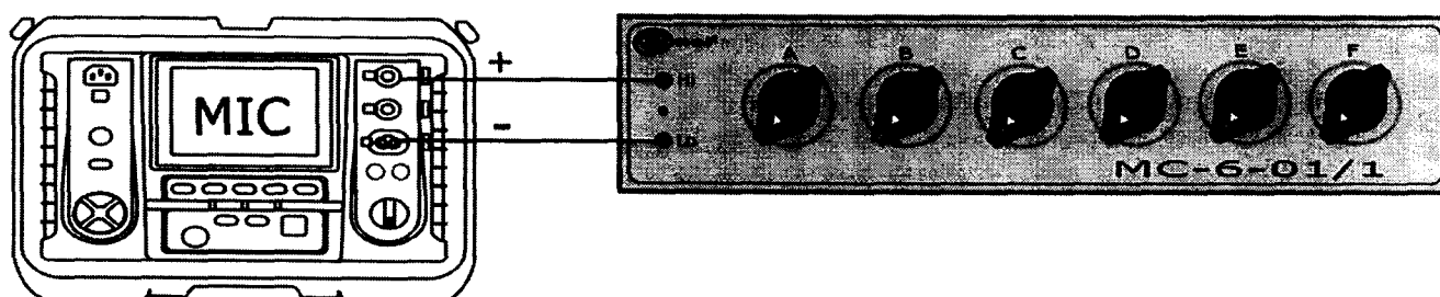
Рисунок 5 - Структурная схема определения абсолютной погрешности измерения сопротивления защитных проводников где MIC – поверяемый измеритель MIC-5010; MC-6-01/1 – магазин электрического сопротивления MC-6-01/1.
