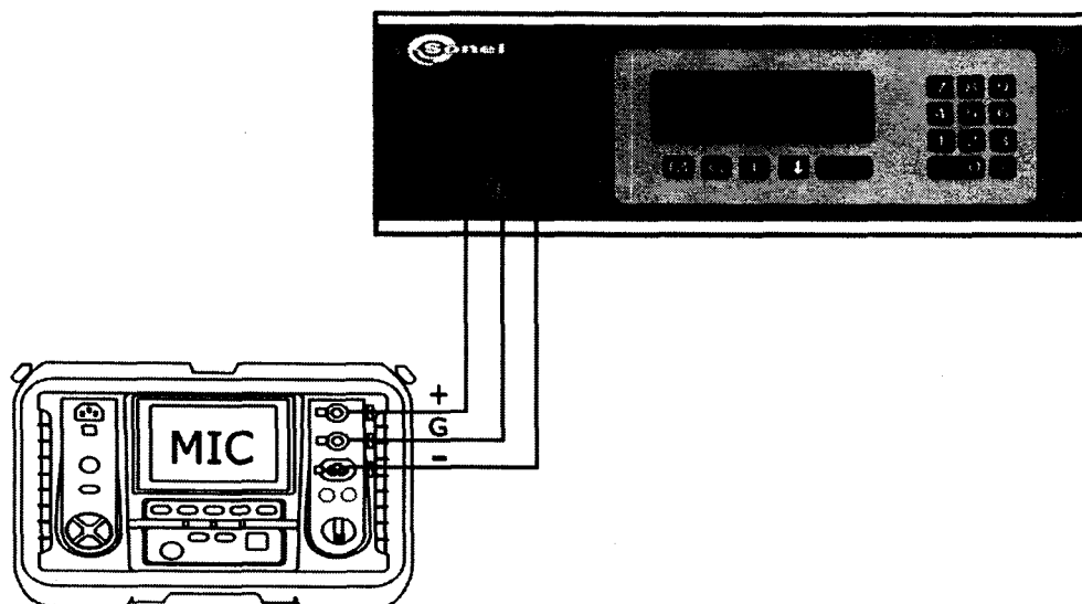
Рисунок 2 - Структурная схема определения абсолютной погрешности измерения сопротивления электроизоляции до 5 ГОм
