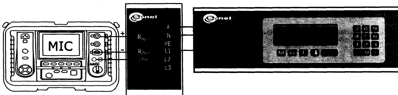
Рисунок 4 - Структурная схема определения абсолютной погрешности измерения сопротивления электроизоляции с адаптером AutoISO-5000 где MIC – поверяемый измеритель MIC-5050, MIC-10k1; KC-100k0-5T0 – калибратор электрического сопротивления KC-100k0-5T0; AutoISO-5000 – адаптер AutoISO-5000.
