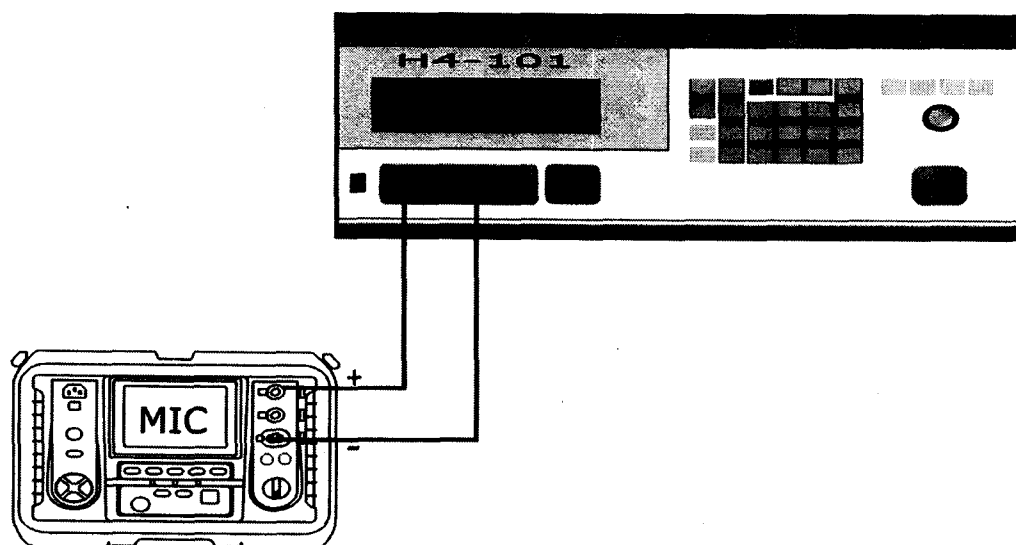
Рисунок 1 - Структурная схема определения абсолютной погрешности измерения напряжения постоянного тока и действующего значения напряжения переменного тока где МІС – поверяемый измеритель МІС-5005, МІС-5010, МІС-5050, МІС-10к1, МІС-15к1; Н4-101 – калибратор универсальный Н4-101.
