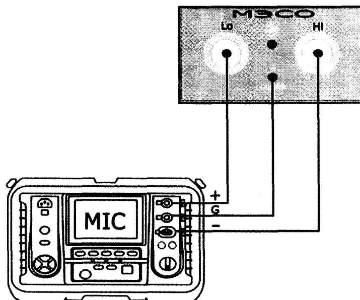
Рисунок 3 - Структурная схема определения абсолютной погрешности измерения сопротивления электроизоляции свыше 5 ТОм где MIC – поверяемый измеритель MIC-5005, MIC-5010, MIC-5050, MIC-10k1, MIC-15k1; МЭСО – меры электрического сопротивления однозначные.
