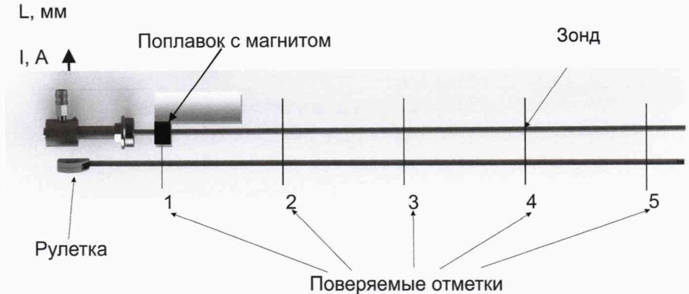
Рисунок 3 – Проверка преобразователя с помощью рулетки и магнитного поплавка
