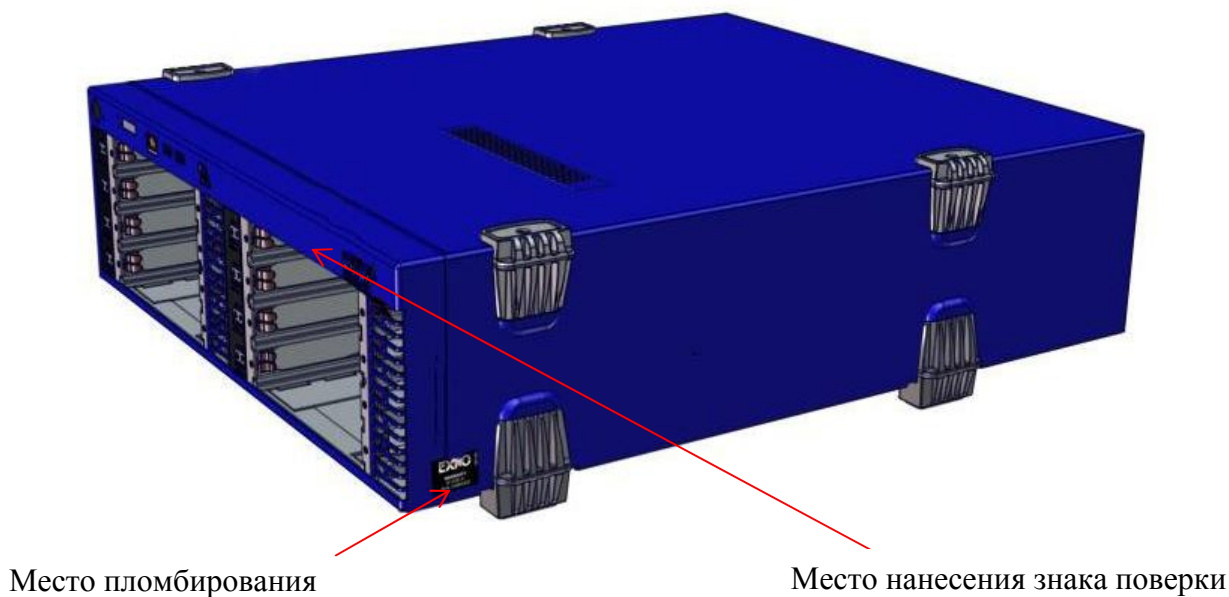
Рисунок 5 – Схема пломбировки системы LTV-8 от несанкционированного доступа, обозначение мест нанесения знака поверки
