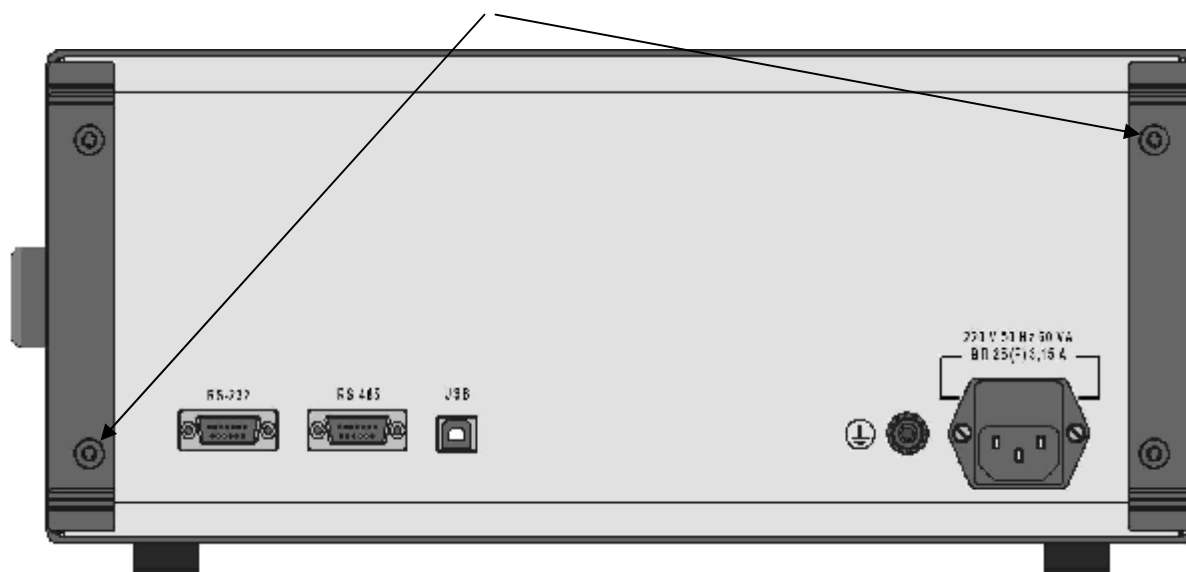
Рисунок 2 – Схема пломбировки от несанкционированного доступа, обозначение мест нанесения знака поверки
