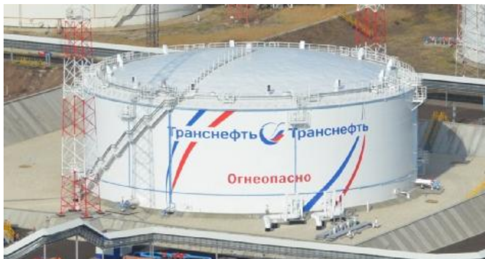
Рисунок 1 – Общий вид резервуаров РВСП-20000 зав.№№ 1, 19, 20, 22
