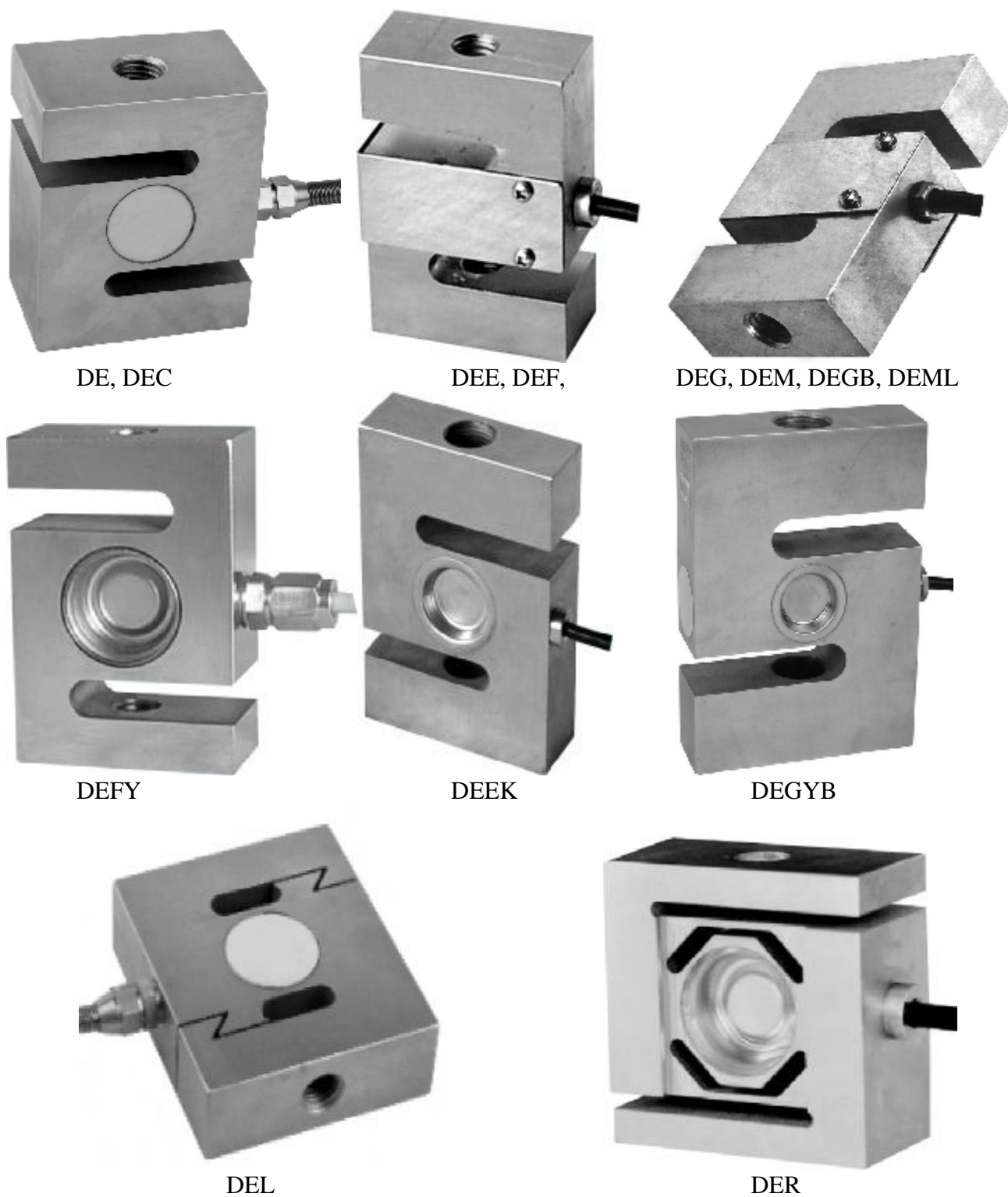
Рисунок 1 — Общий вид средства измерений (примеры)
