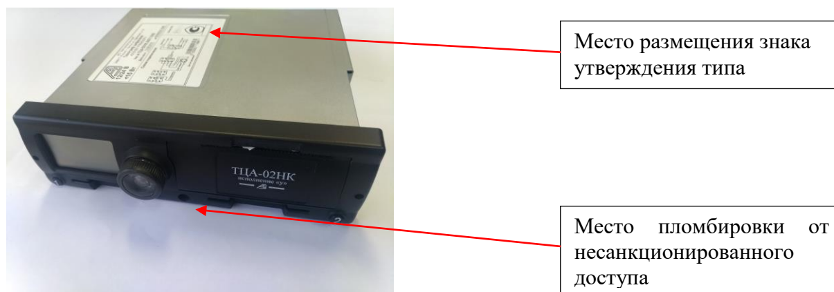
Рисунок 2 – Место размещения знака утверждения типа и схема пломбировки от несанкционированного доступа
