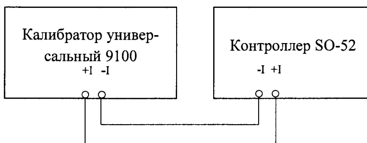
Рисунок 4 – Схема подключения при измерении силы постоянного тока
