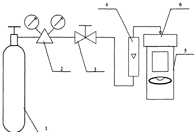
Рисунок 1 – Схема подачи ПГС в ИК системы измерительной газоаналитической модели MeshGuard SS
