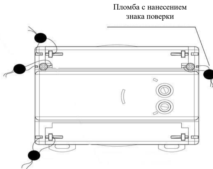
а) счетчики в корпусе 9МТН35
