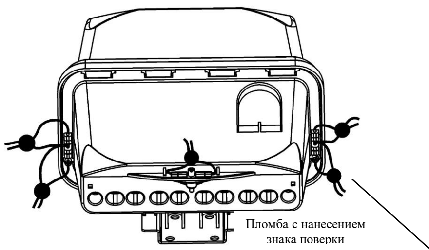
в) счетчики в корпусе SPLIT
