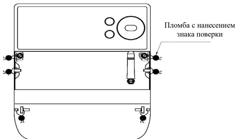
б) счетчики в корпусе 10м
