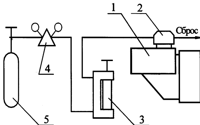
Рисунок В.1 – Рекомендуемая схема подачи ГС на вход газоанализаторов 1 – газоанализатор; 2 – насадка; 3 – ротаметр РМ-А-0,063, 4 – редуктор (регулятор расхода поверочной газовой смеси) 5 – баллон с поверочной газовой смесью.
