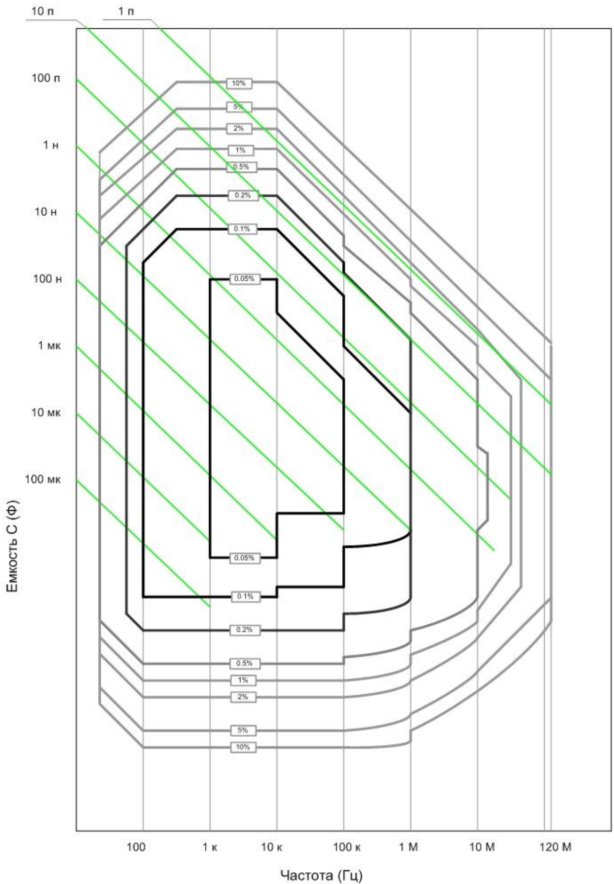
Рисунок 2. График зависимости погрешности (от 0,05 до 10) % измерения емкости от номинального значения и частоты
