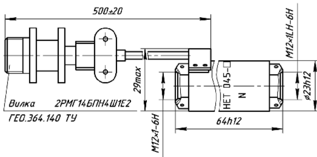
Рисунок 2 – Габаритные и установочные размеры датчика силы HET 045
