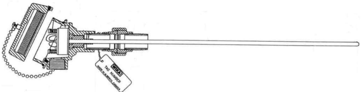
Рис. 1. Чертеж термопреобразователя.
