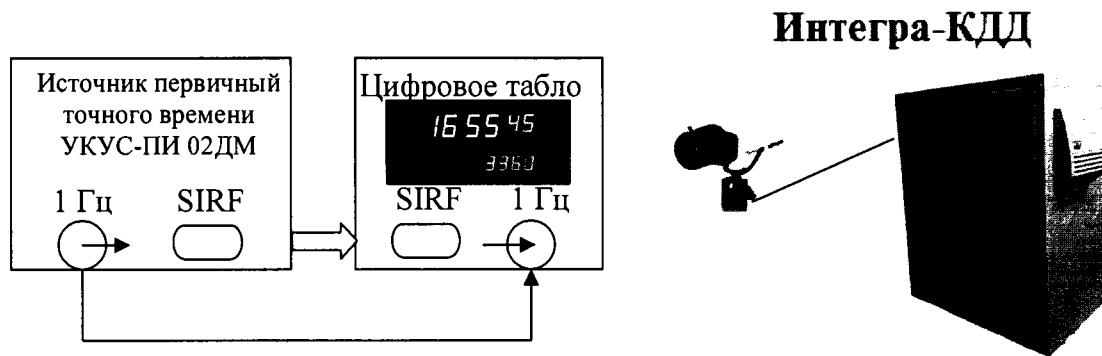
Рисунок 2 – Схема определения пределов допускаемой абсолютной погрешности привязки текущего значения времени к шкале времени UTC (SU).
