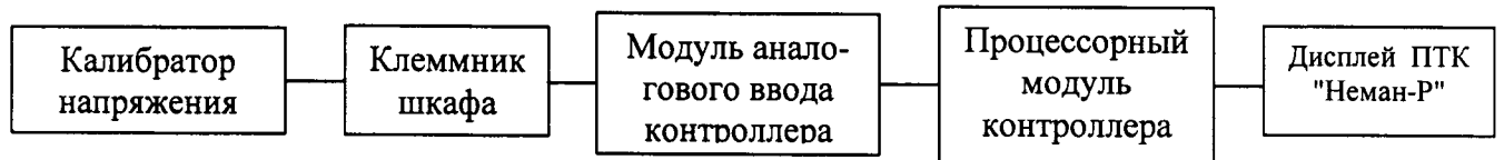
Рисунок 4 - Структурная схема поверки АИК, работающего с вторичными преобразователями с выходом 0...10 В, ±10 В
