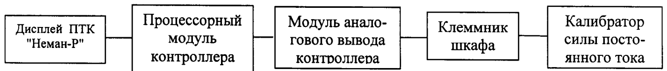
Рисунок 6 - Структурная схема поверки АУК, с унифицированным выходом 4...20 мА
