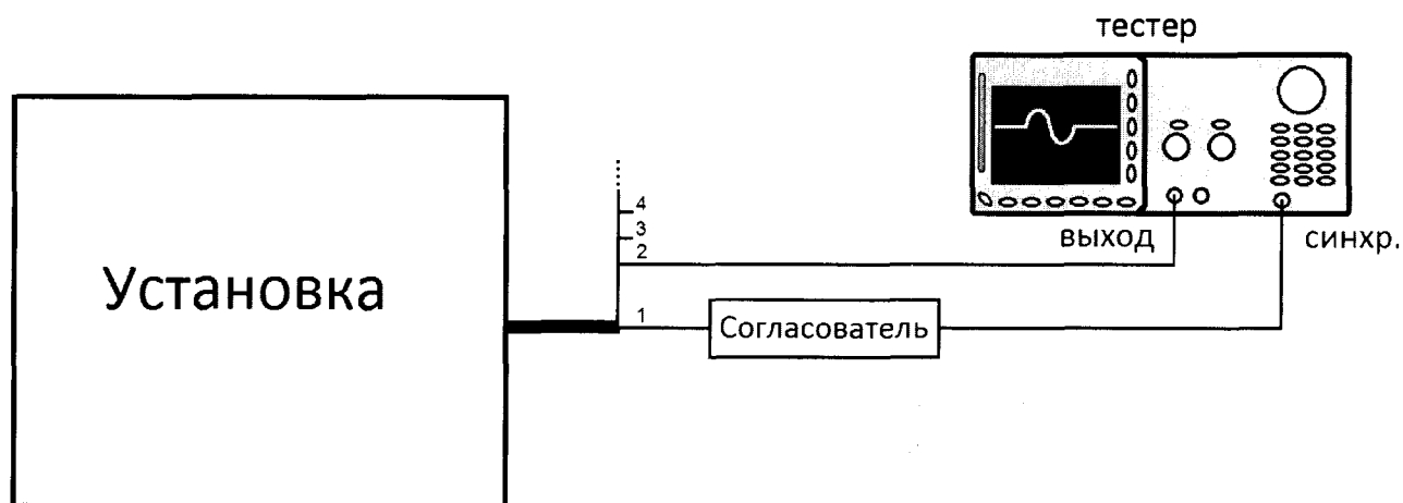
Рисунок 6 – Схема соединения
