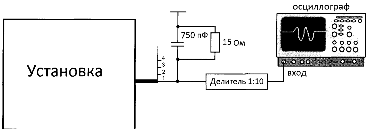
Рисунок 1 – Схема соединения
