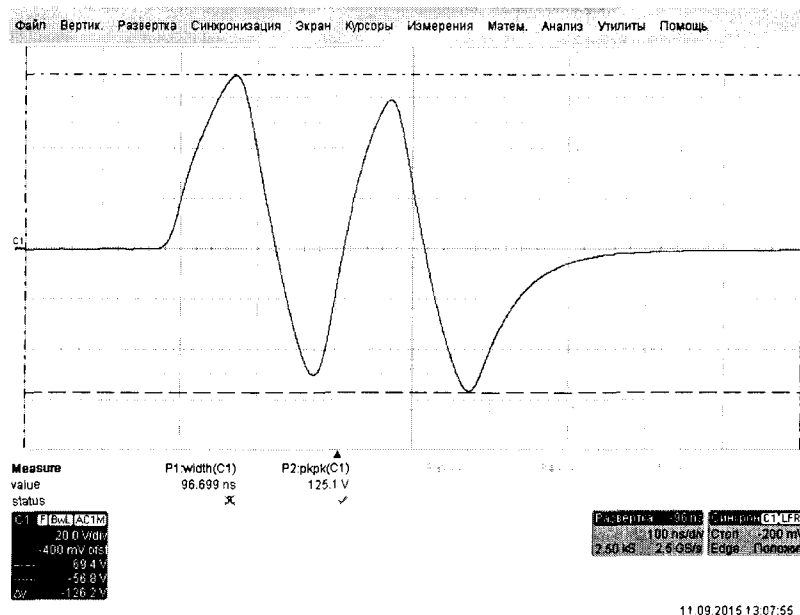
Рисунок 2 – Экран осциллографа при измерении амплитуды импульсов ГИВ
