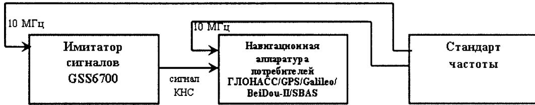
Рисунок 4 – Схема измерений для определения погрешности формирования беззапросной дальности
