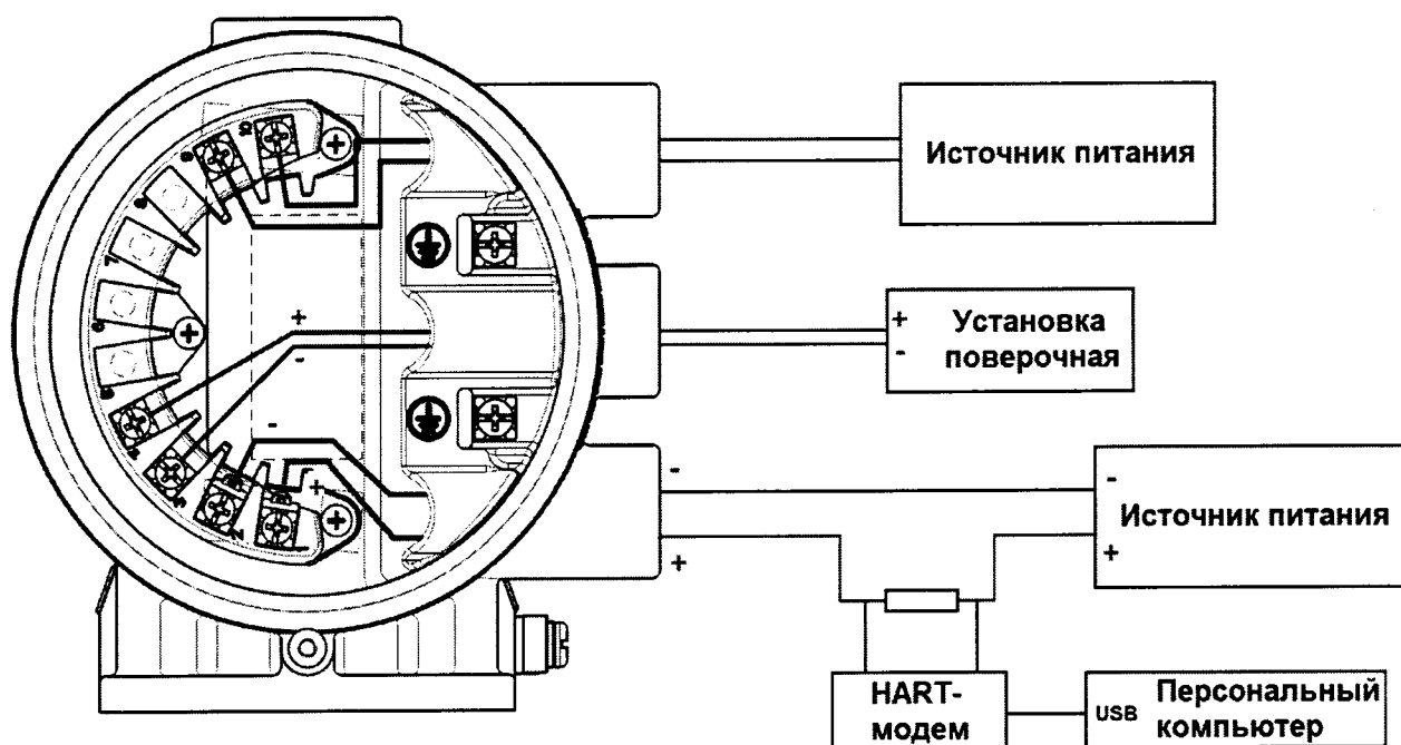
Рисунок А.2 – Схема подключения расходомера при определении погрешностей измерения объема или объемного расхода с использованием сервисного ПО AMS, Prolink
