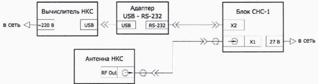
Рисунок 1 — Схема подключения наземной части ИИС-32М для проверки работоспособности
