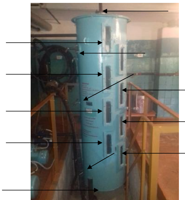
Рисунок 1 - Общий вид и места пломбирования мерника
