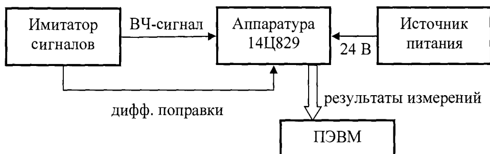
Рисунок 1 - Схема измерений
