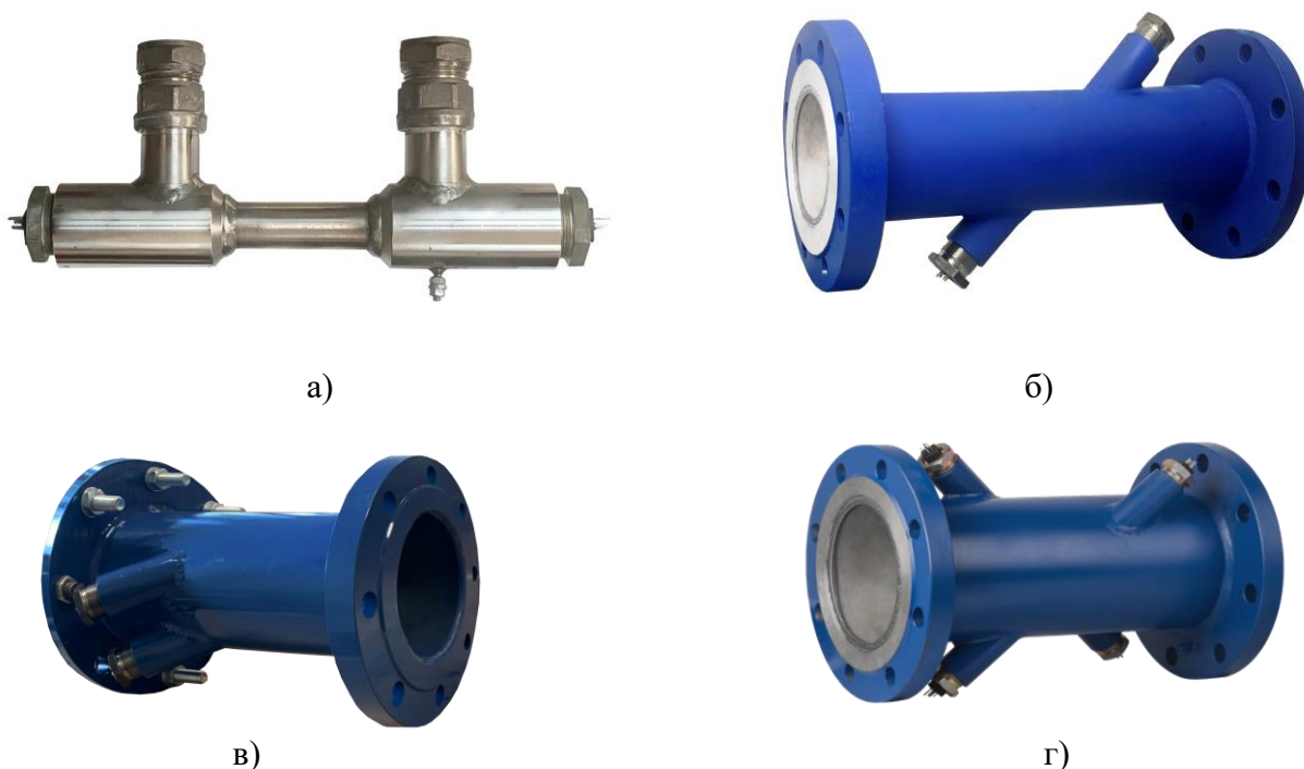
Рисунок 2 – Варианты исполнений УПР: а) – исполнение УПР с U-образным ИУ; б) – исполнение УПР с прямым ИУ по однолучевой схеме с диаметральной расположением акустического канала; в) – исполнение УПР с прямым ИУ по двухлучевой схеме с расположением акустических каналов на параллельных хордах г) – исполнение УПР с
