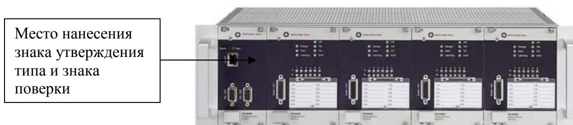
Рисунок 1- Внешний вид аппаратуры измерения параметров вибрации многоканальная VC-6000
