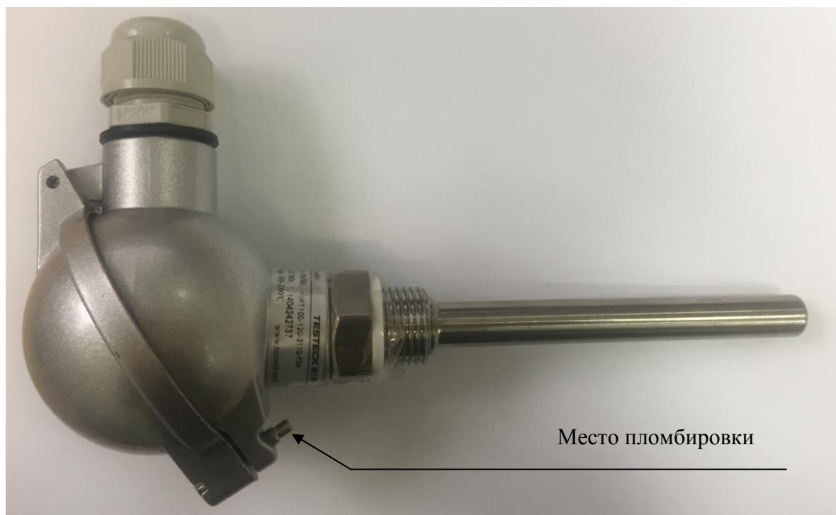
Рисунок 1 - Общий вид термопреобразователя сопротивления платинового LF12Pt100-120-3110-F04
