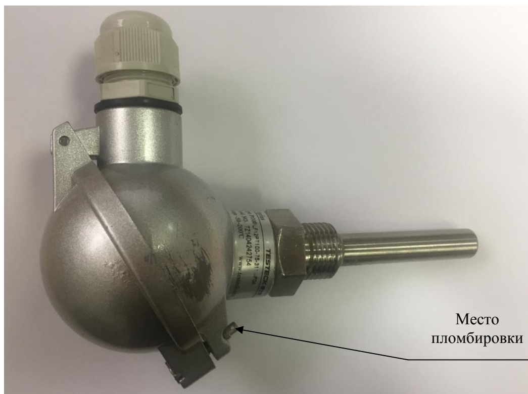
Рисунок 1 - Общий вид термопреобразователя сопротивления платинового LF12PT100-75-3110-F04
