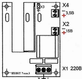
Рис. Н.1 Внешний вид БП/ВКТ-7
