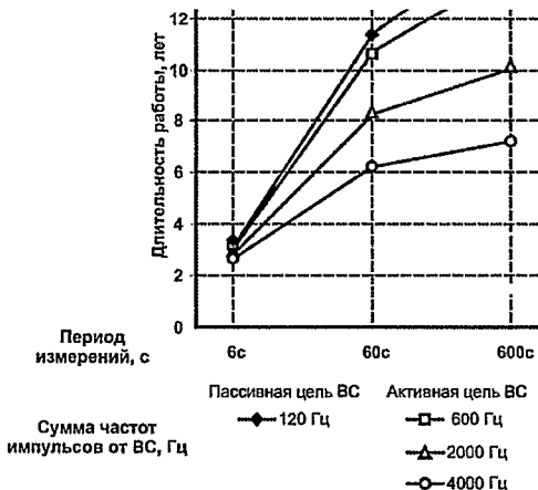
Рис. 2.1 – Зависимость ресурса батареи ВКТ-7М
