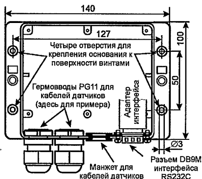
Рис. 6.1—Схема крепления корпуса ВКТ-7М
