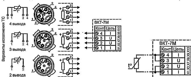
а) Подключение ТС по 4-проводной схеме
