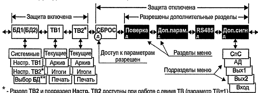
Рис. 3.5 – Структура меню вычислителя
