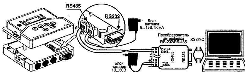
Рис. Д3 – Схема подключения адаптера интерфейса RS 485
