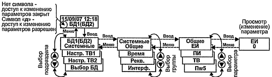
Рис. 4.1 – Пример просмотра значения параметра ЕИ
