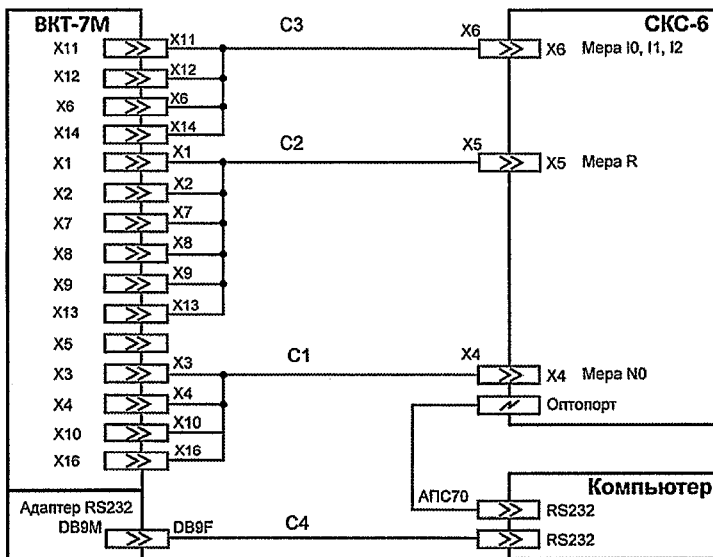
Рисунок 8.1 – Схема поверки
