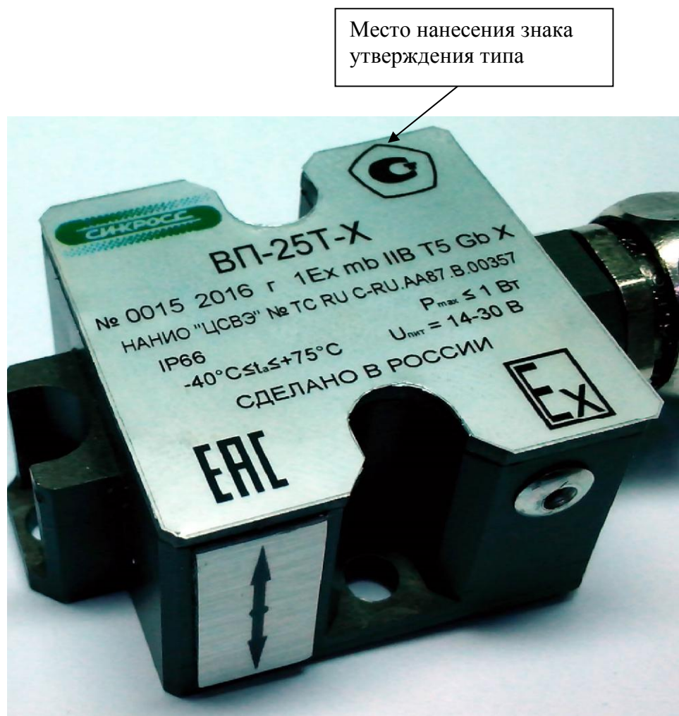
Рисунок 1- Внешний вид вибропреобразователя ВП-25Т
