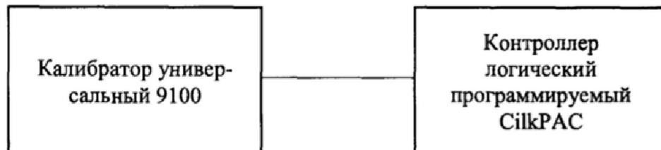
Рисунок 1 – Структурная схема проверки допускаемой погрешностей контроллера
