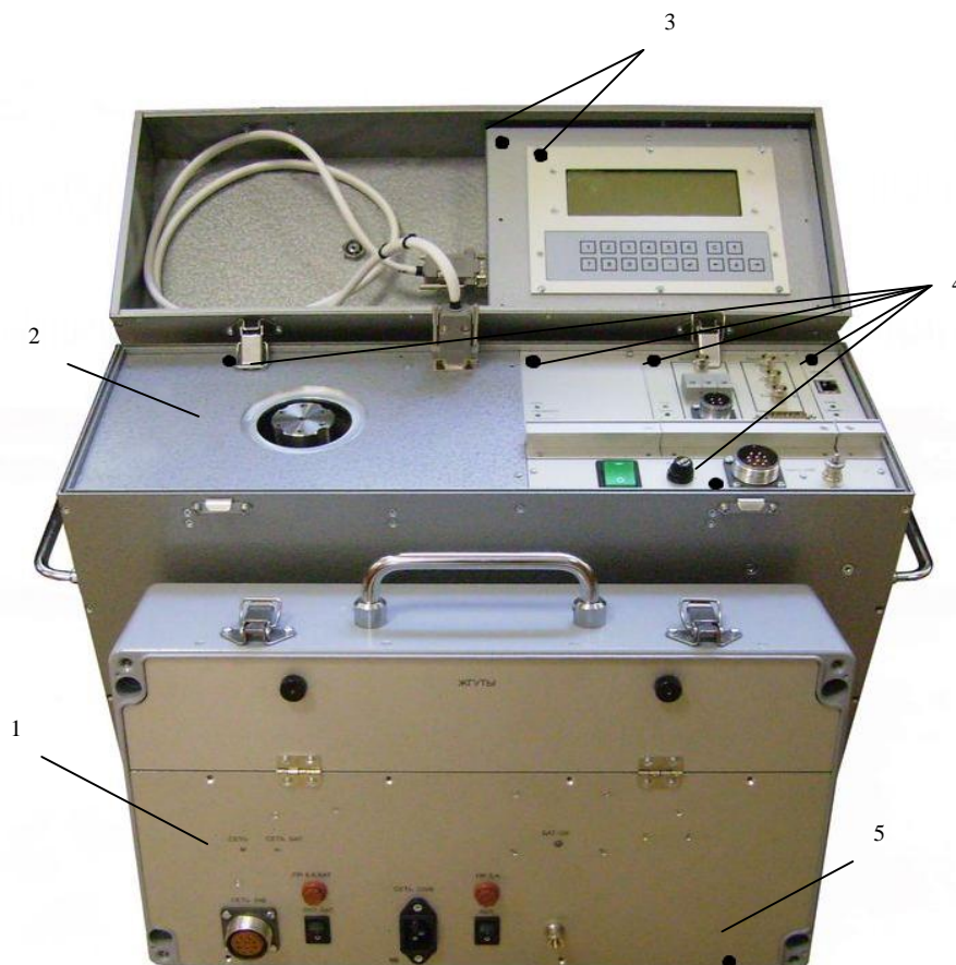
Рисунок 1 – Общий вид установки вибрационной поверочной ВМВП
