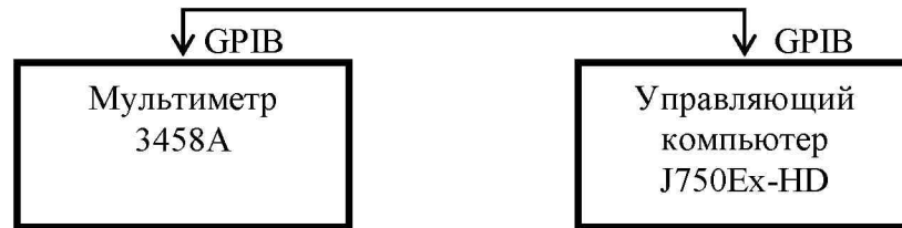
Рисунок 1 – Схема подключения кабеля GPIB для калибровки модуля «CAL-CUB»
