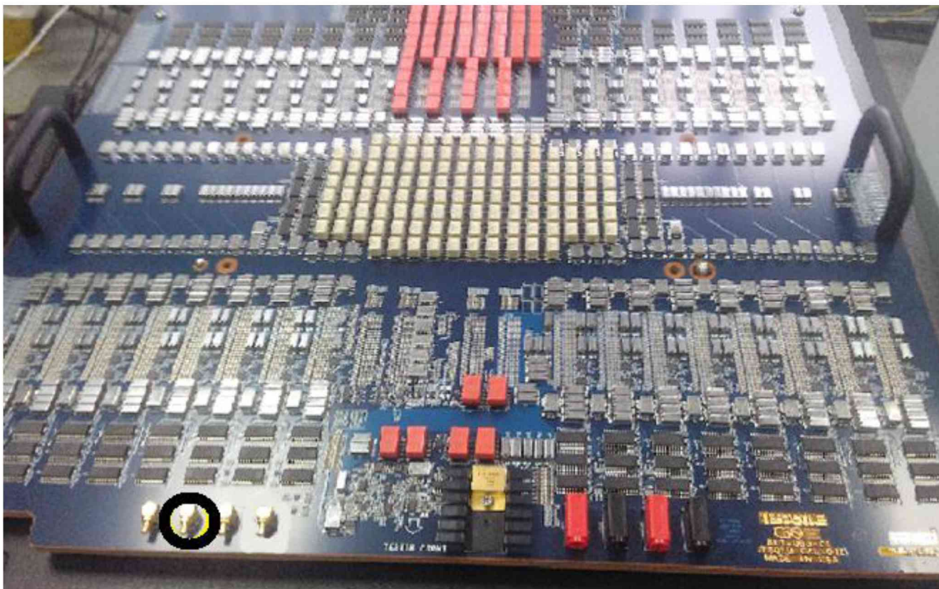
Рисунок 7 – Расположение разъема CLK_N на плате CAL-DIB
