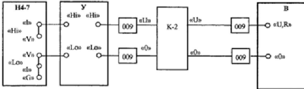
Рисунок 5.1 - Схема соединения приборов для определения погрешности вольтметра при измерении напряжения постоянного и переменного токов на диапазонах с верхними пределами измерений U_k 200 мВ; 2; 20 В, напряжения постоянного тока на диапазоне с верхним пределом измерения U_k 200 В.
