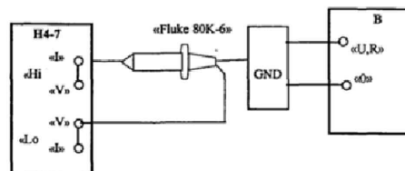
Н4-7 - калибратор универсальный; В - поверяемый вольтметр; Fluke 80K-6, GND - щуп высоковольтный из комплекта поверяемого вольтметра.
