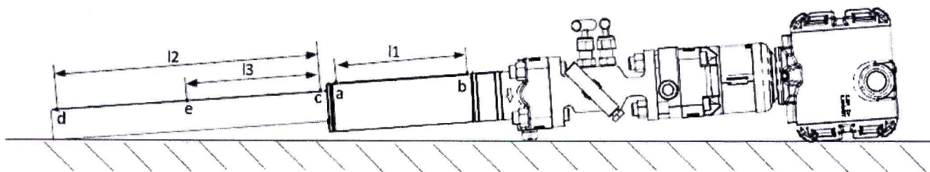
Рисунок А.2. – Схема измерений отклонения от прямолинейности ОНТ
