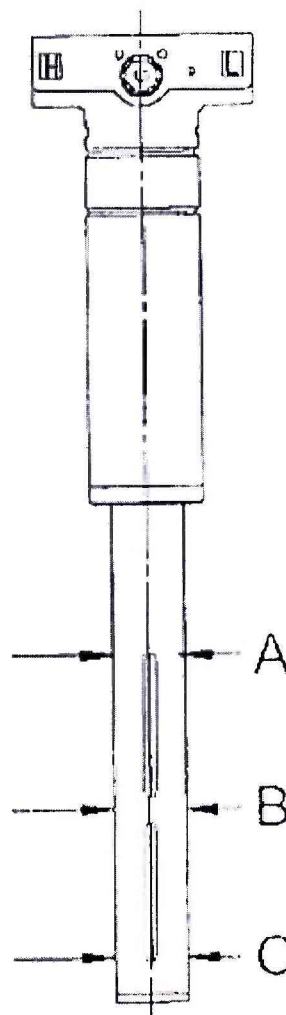
Рисунок А.1. – Схема измерений линейных размеров ОНТ
