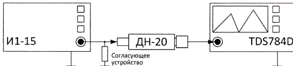
Рисунок 1 – Схема измерений при опробовании и определении коэффициента преобразования делителя
