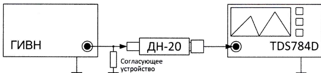
Рисунок 2 – Схема измерений при определении коэффициента преобразования делителя
