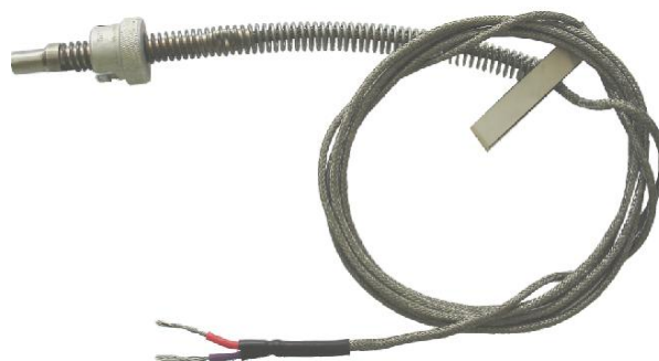
Рисунок 2 - Внешний вид преобразователей термоэлектрических ТЖК(Ж)-1199, ТХА(К)-1199, ТХК(Л)-1199, ТНН(Н)-1199 исполнения 46
