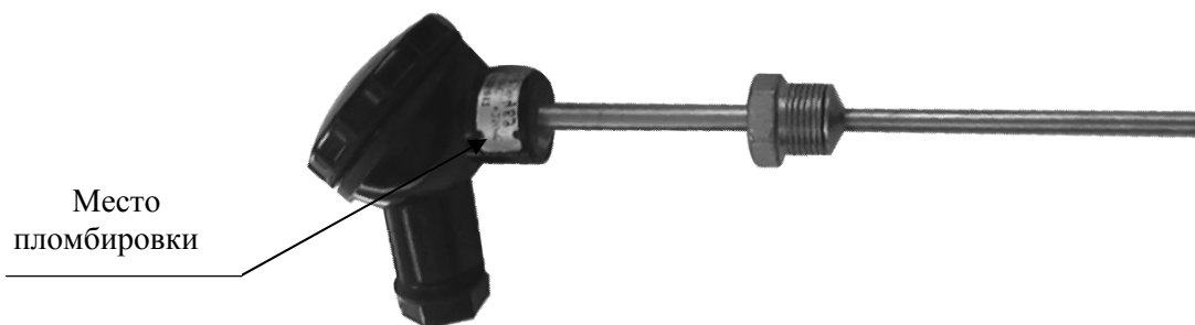
Рисунок 1 - Внешний вид преобразователей термоэлектрических ТЖК(Ж)-1199, ТХА(К)-1199, ТХК(Л)-1199, ТНН(Н)-1199 исполнения 11
