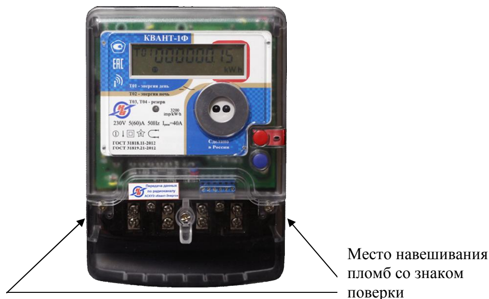
Рисунок 1 - Внешний вид счетчика электрической энергии однофазного многотарифного «КВАНТ-1Ф» с местами опломбирования и нанесения знака поверки
