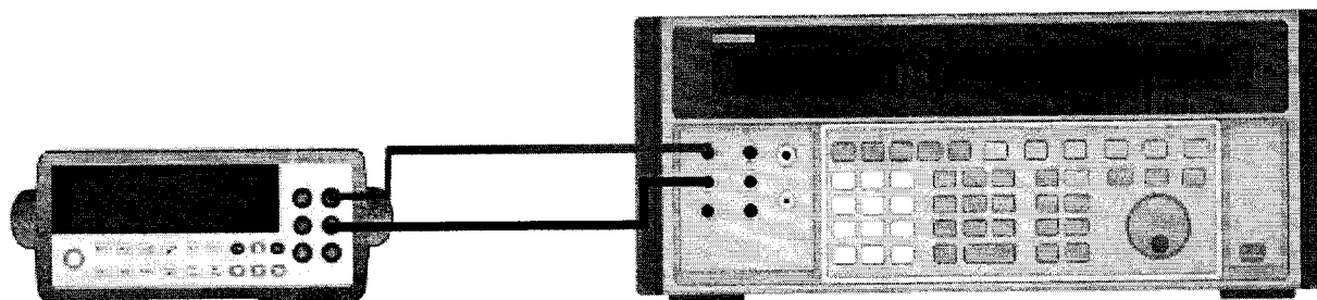
Рисунок 6 – Двухпроводная схема измерений без компенсации (для диапазона 1 – 100 МОм)
