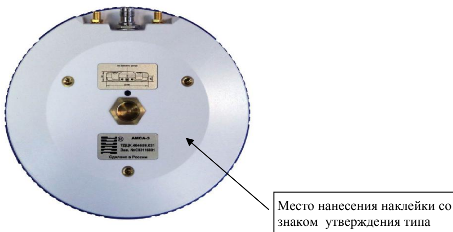
Рисунок 3 – Внешний вид модуля антенного гибридного ГНСС со стороны нижней панели
