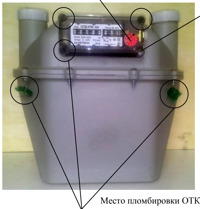
Рисунок 2 – Схема опломбирования счетчика, обозначение мест нанесения знака поверки
