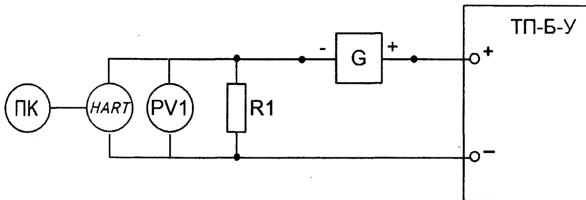
Рисунок Г.1 - Схема подключения внешних цепей ТП-Б-У с выходным сигналом от 4 до 20 мА
