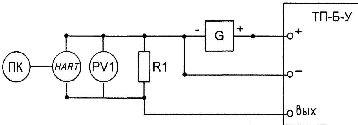
Рисунок Г.2 - Схема подключения внешних цепей ТП-Б-У с выходным сигналом от 0 до 20 мА и от 0 до 5 мА
