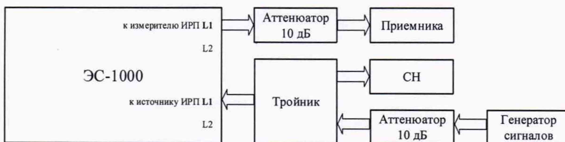
Рисунок 2 - Схема измерений выходного уровня эквивалента сети
